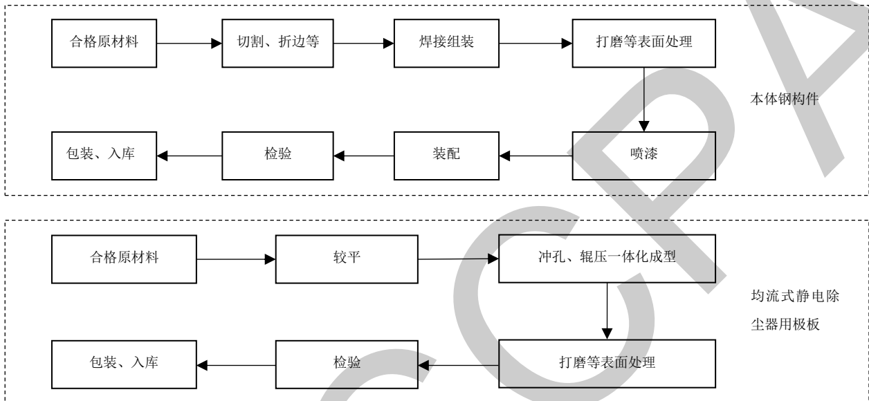
图 A.2 均流式电除尘器工艺流程图
