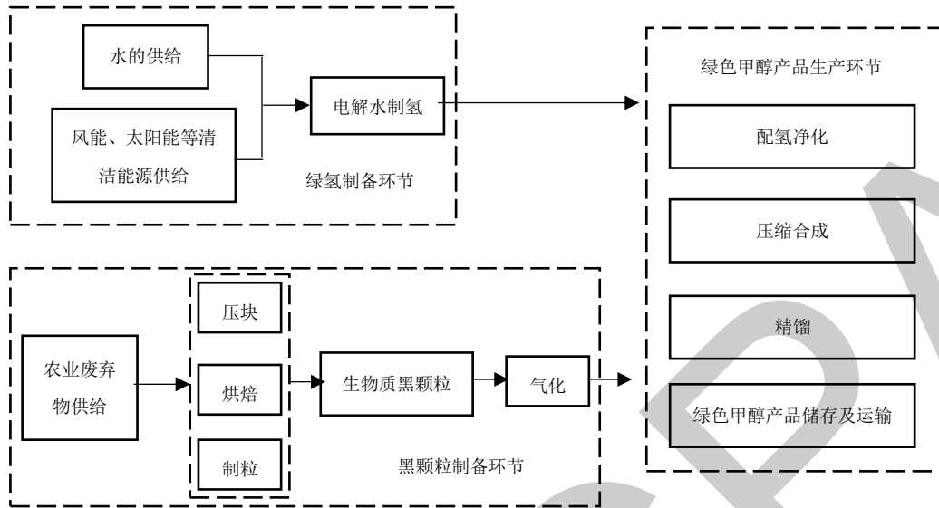
图 1 绿色甲醇产品生命周期系统边界
