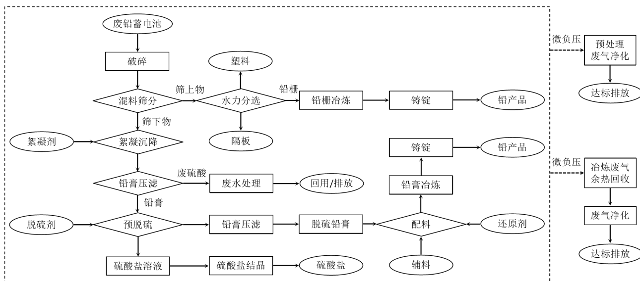
图 1 废铅酸蓄电池破碎分选-铅膏预脱硫-铅冶炼工艺路线
